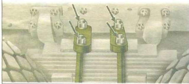
Рис. 23. Закрепить стремянки задних рессор.
