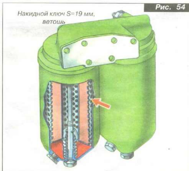
Рис. 54. Сменить фильтрующие элементы масляного фильтра.
