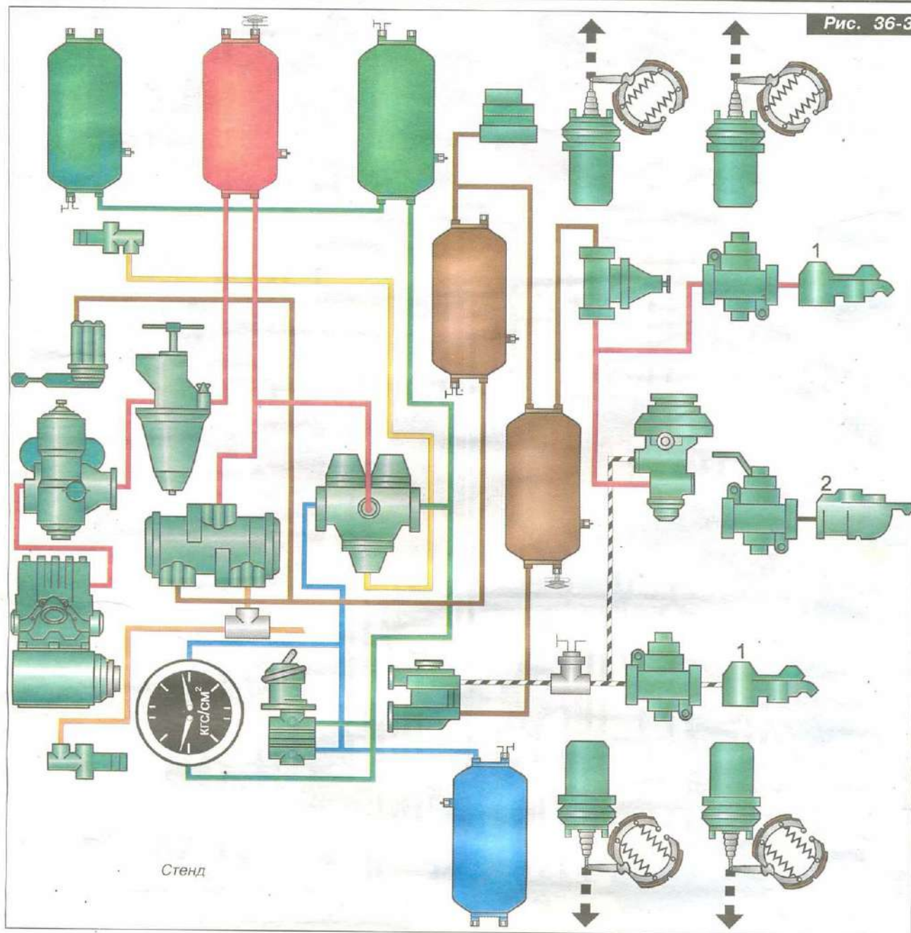
Рис. 36-3. Установить рукоятку крана управления стояночной тормозной системой в вертикальное фиксированное положение.
