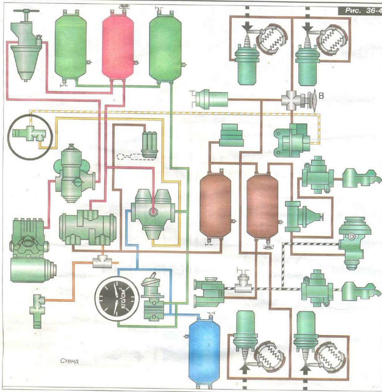
Рис. 36-4. Когда рукоятка крана управления стояночной тормозной системой находится в вертикальном фиксированном положении, нажать кнопку крана аварийного растормаживания.
